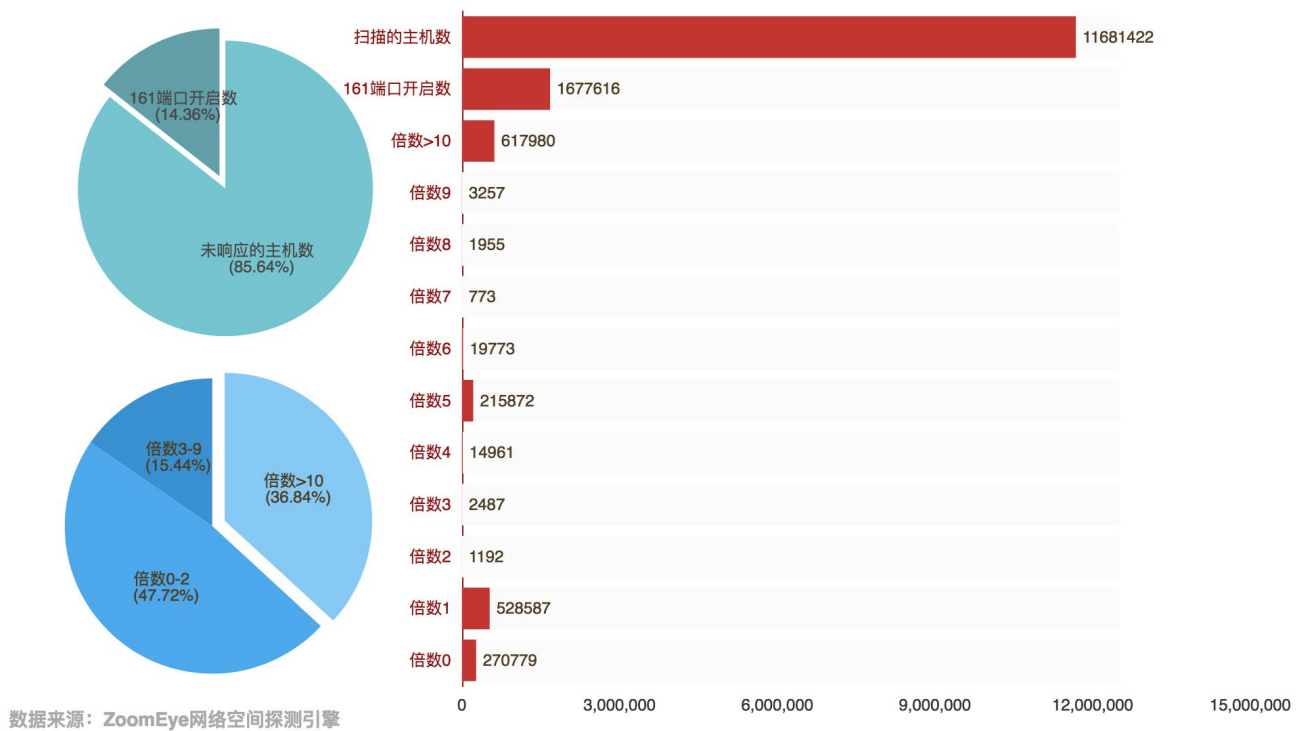
3.4-1 SNMP协议161端口探测统计图
